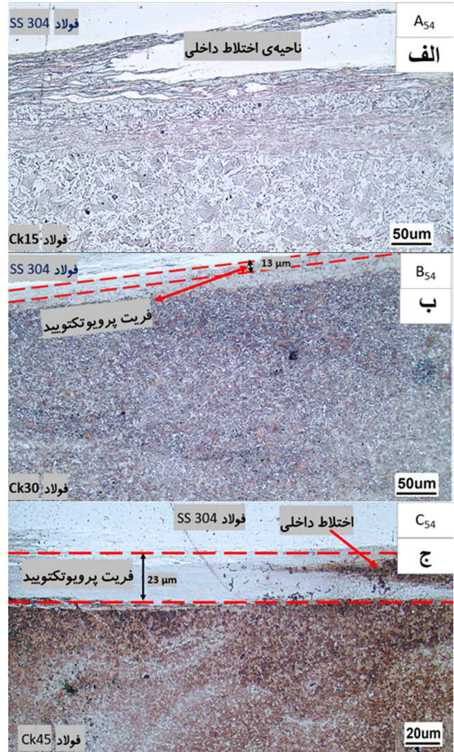
شکل 8- تصاویر میکروسکوپ نوری از ریزساختار ناحیه جوش سه نمونه الف - A 54 ، ب - B 54 و ج - C 54 در سمت ساده کربنی.
